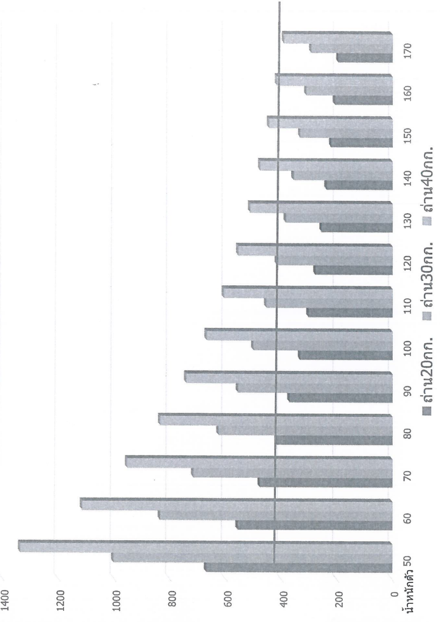
ตารางเปรียบเทียบน้ำหนักตัว ต่อ ปริมาณเชื้อเพลิง (ถ่านไม้) และอุณหภูมิการเผาไหม้
